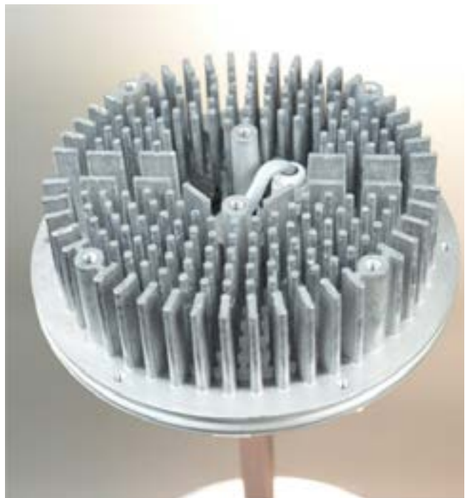
Ein speziell entwickelter Kühlkörper für flexible Einbausätze
